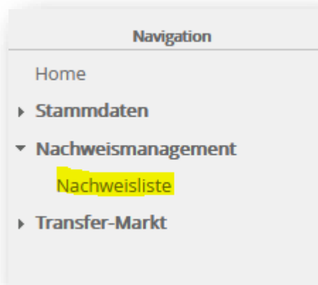
Abbildung 21: Navigation Nachweisliste
