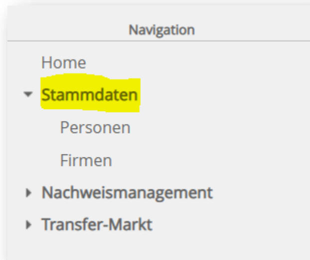
Abbildung 14: Auswahl Stammdaten
