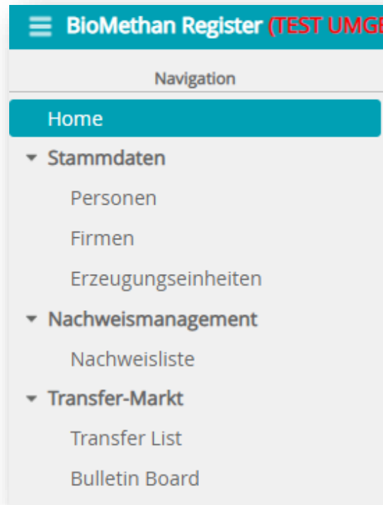
Abbildung 4: Ansicht „Navigation“
